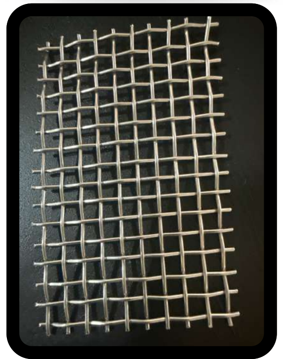
MESH 6X6 CAL 20 ABERT 3.353 MM
