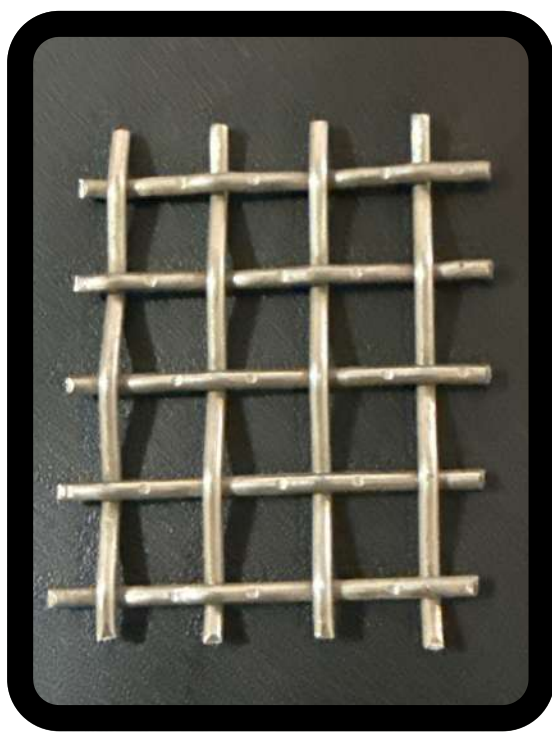
MESH 3X3 CAL 16 ABERT 6.858 MM
