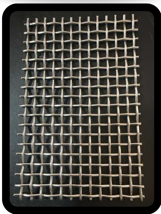
MESH 8X8 CAL 21 ABERT 2.362 MM
