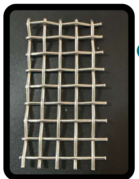
MESH 4X4 CAL 18 ABERT 5.156MM
