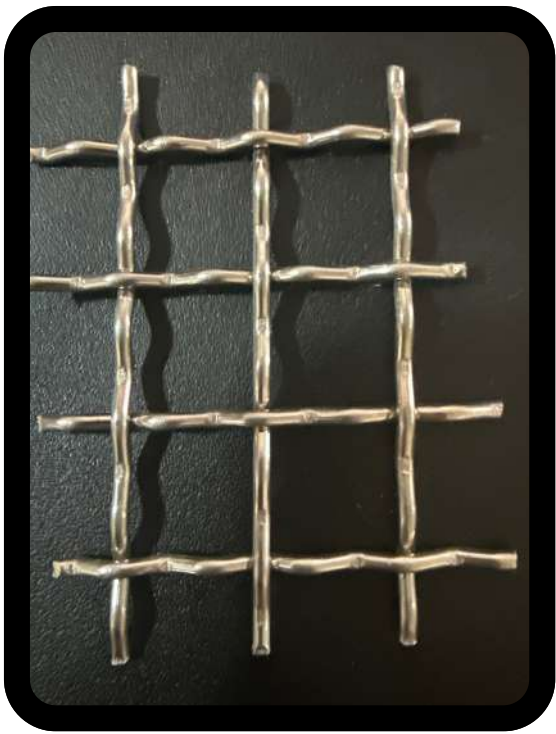
MESH 2X2 CAL 16 ABERT 11.100 MM
